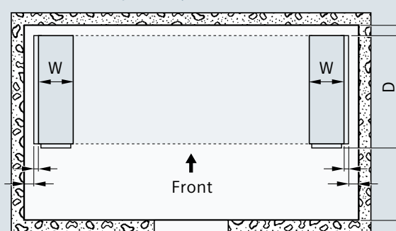
Planificación de compartimento (altura de compartimento \geq 2,850 mm) Conexión frontal
